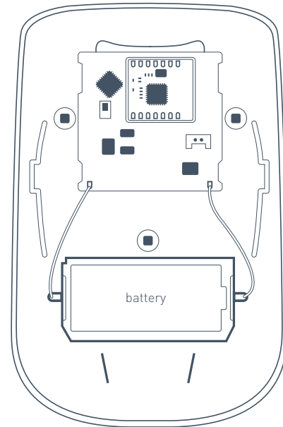
РИС. 5. Вид датчика со снятой верхней крышкой
