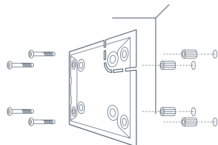
РИС. 2. Схема монтажа крепежной панели SmartBracket
